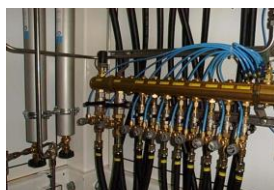
Medienverteilung für Kühlwasser, CDA, Stickstoff
